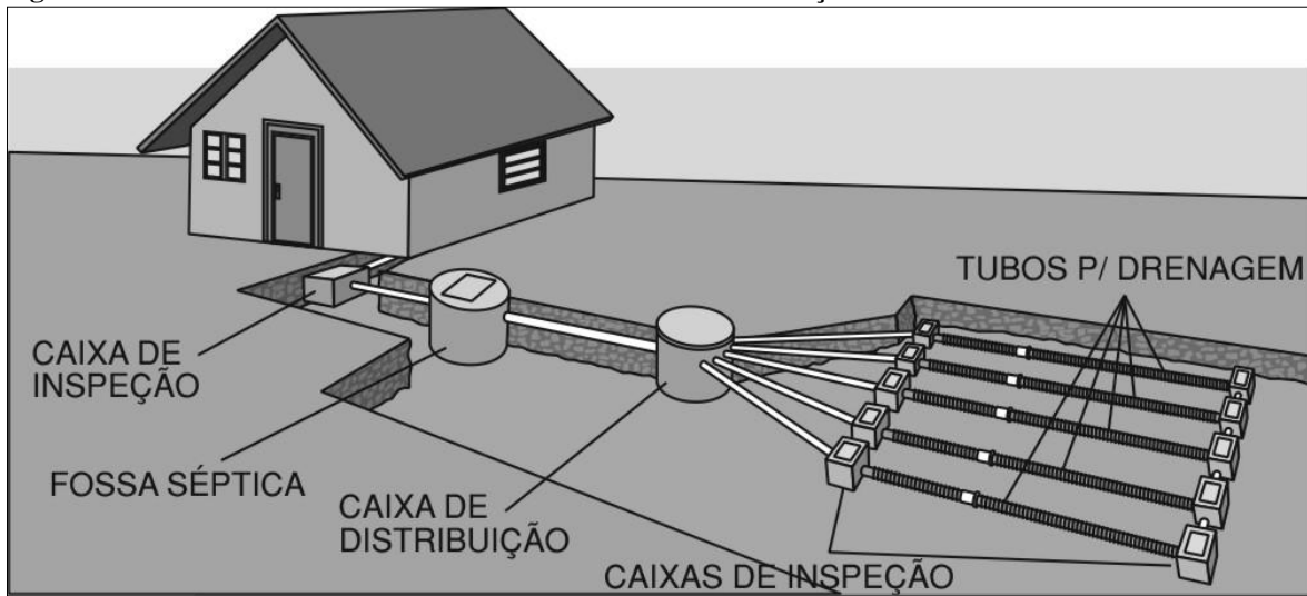
Figura 40 - Sistemas de tratamento individual– Valas de Infiltração.
