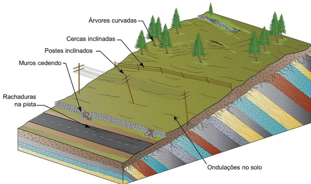
Figura 60 – Esquema do movimento de massa do tipo Rastejo.
