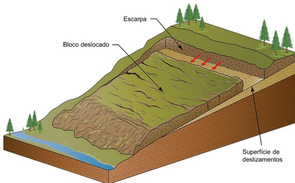
Figura 61 – Esquema dos escorregamentos planares ou translacionais.
