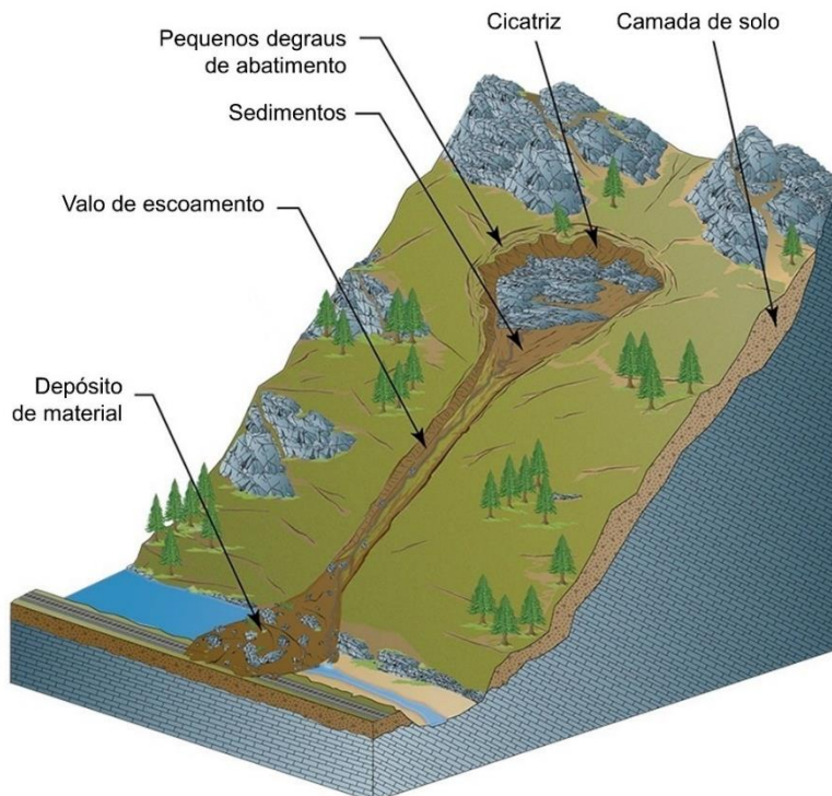
Figura 64 – Esquema do movimento de massa do tipo corrida.
