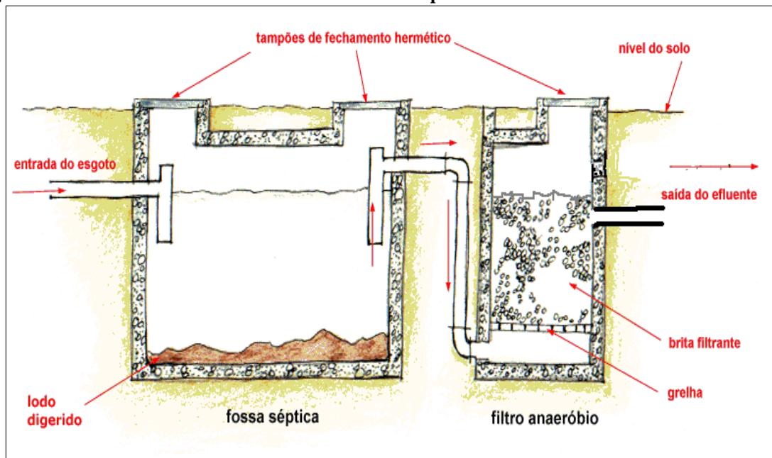
Figura 39 - Sistema individual de tratamento - Fossas Sépticas.
