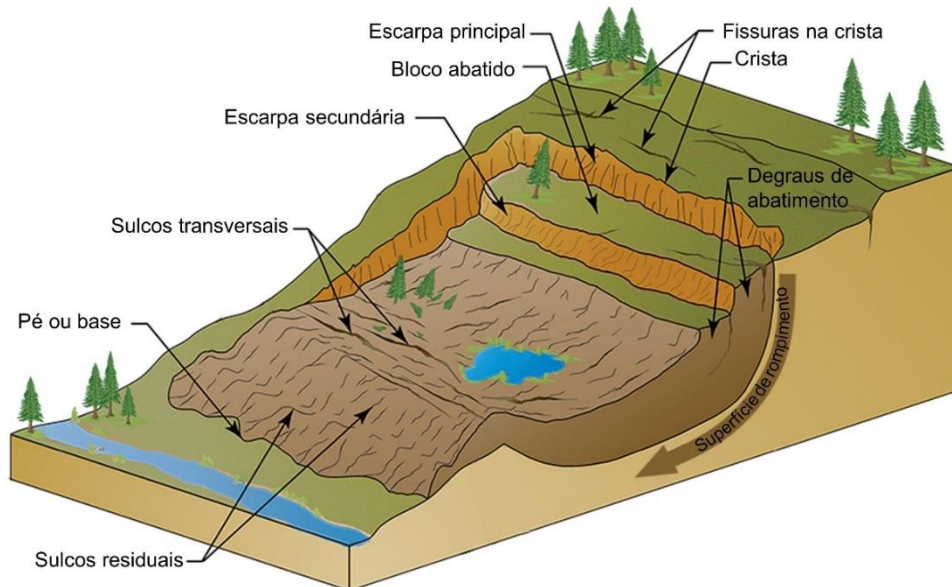
Figura 62 – Esquema dos escorregamentos circulares ou rotacionais.
